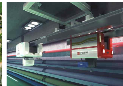
管廊机器人
